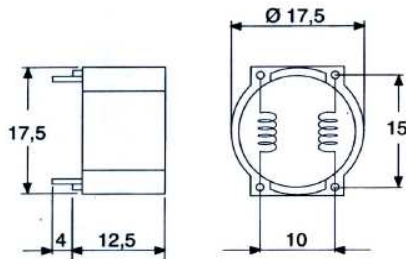
2 : Boîtier Horizontal / Horizontal case
