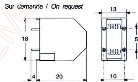
1 : Boîtier Vertical / Vertical case
