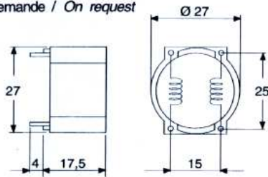
2 : Boîtier Horizontal / Horizontal case
